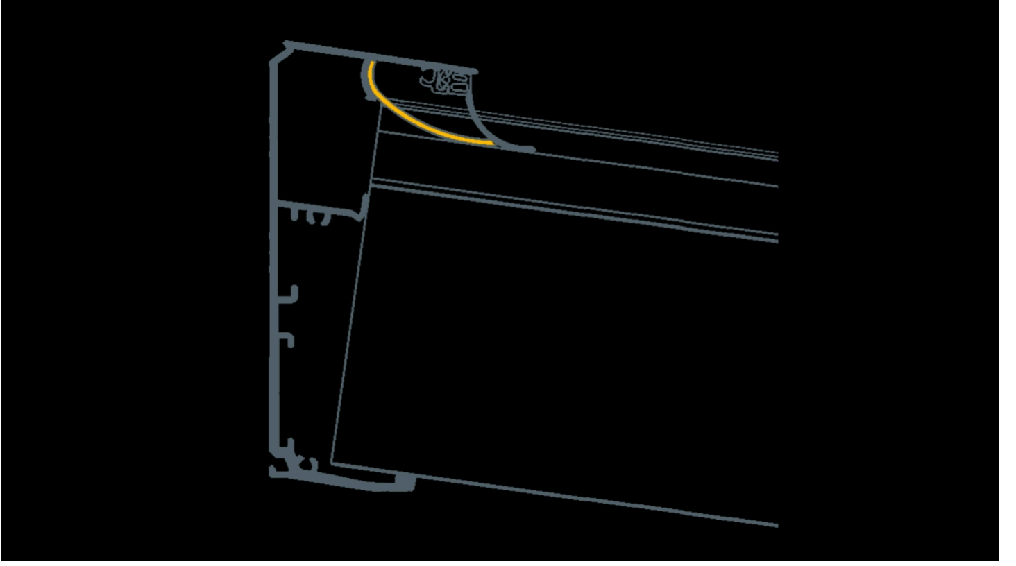
İzoflex duvar yalıtım membranı ile çift katmanlı su yalıtımı
